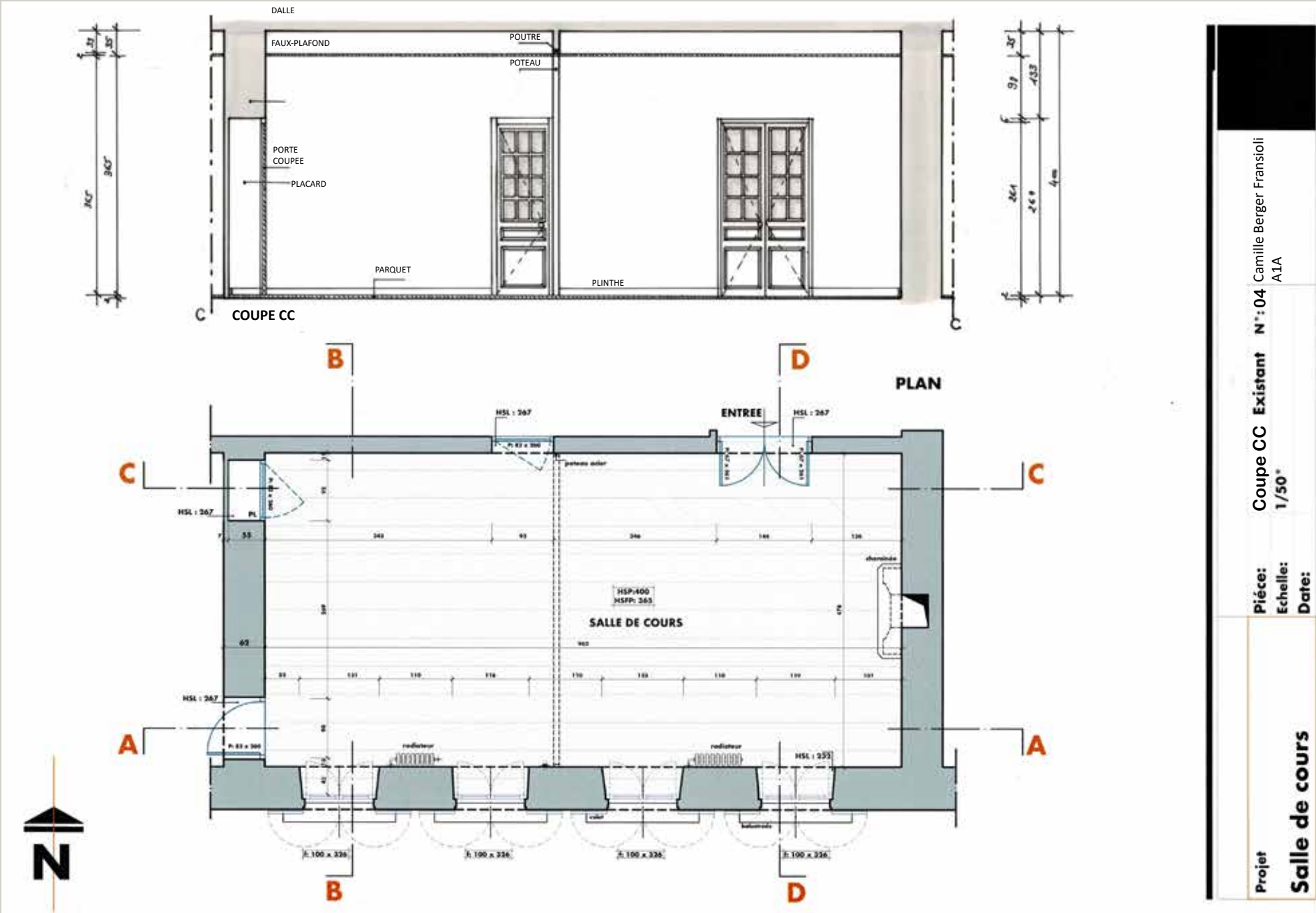
Salle de cours - Coupe CC réalisée au 1:50. Présentation Echelle N/C.
