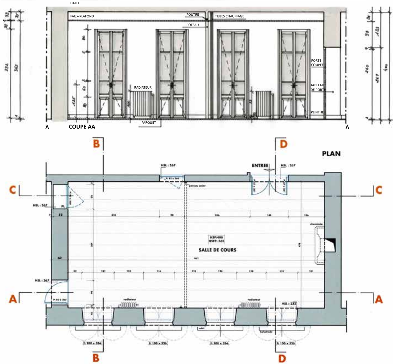
Salle de cours - Coupe AA réalisée au 1:50. Présentation Echelle N/C.
