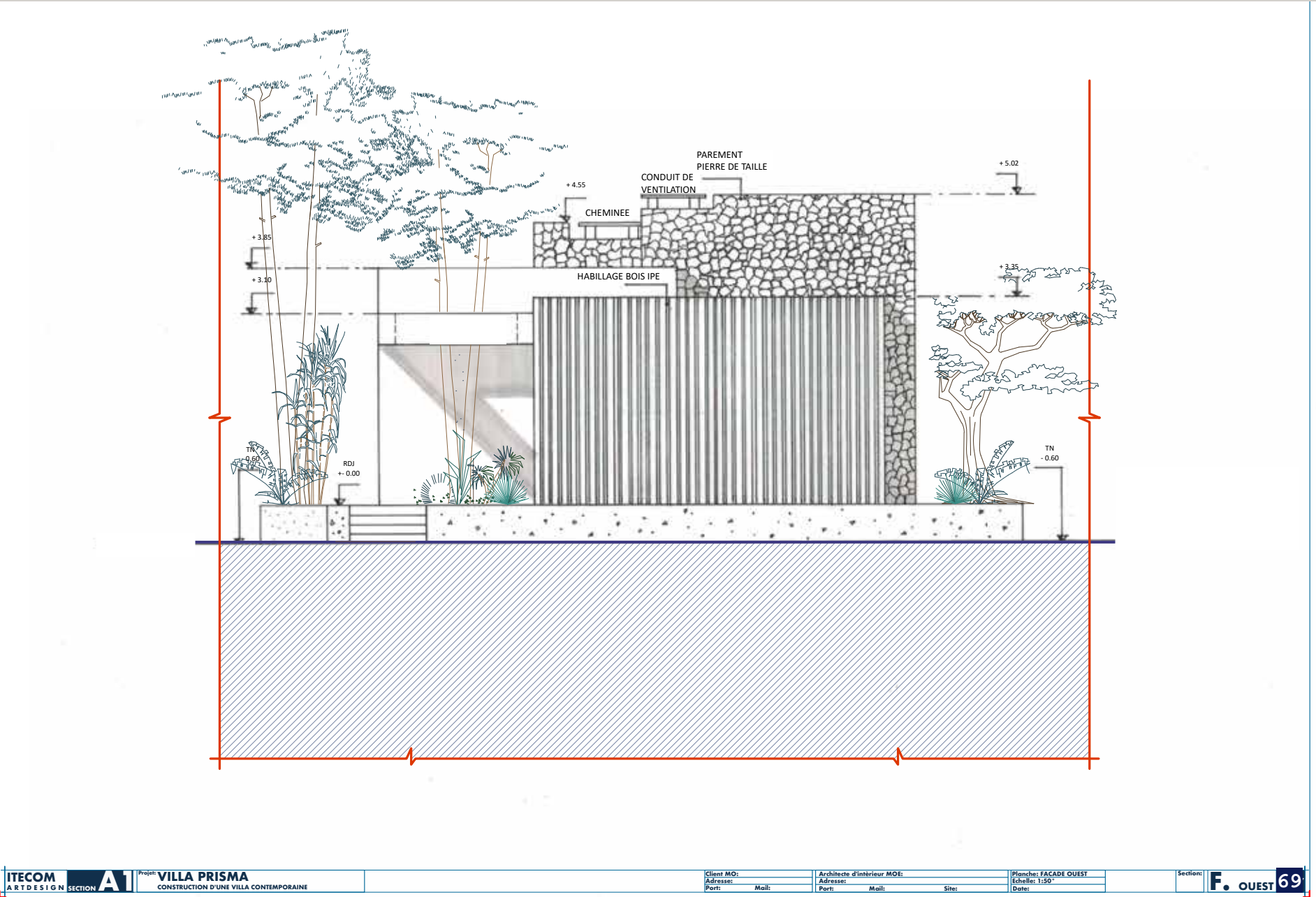
Villa Prisma - Façade Ouest réalisée au 1:50. Présentation Echelle N/C.
