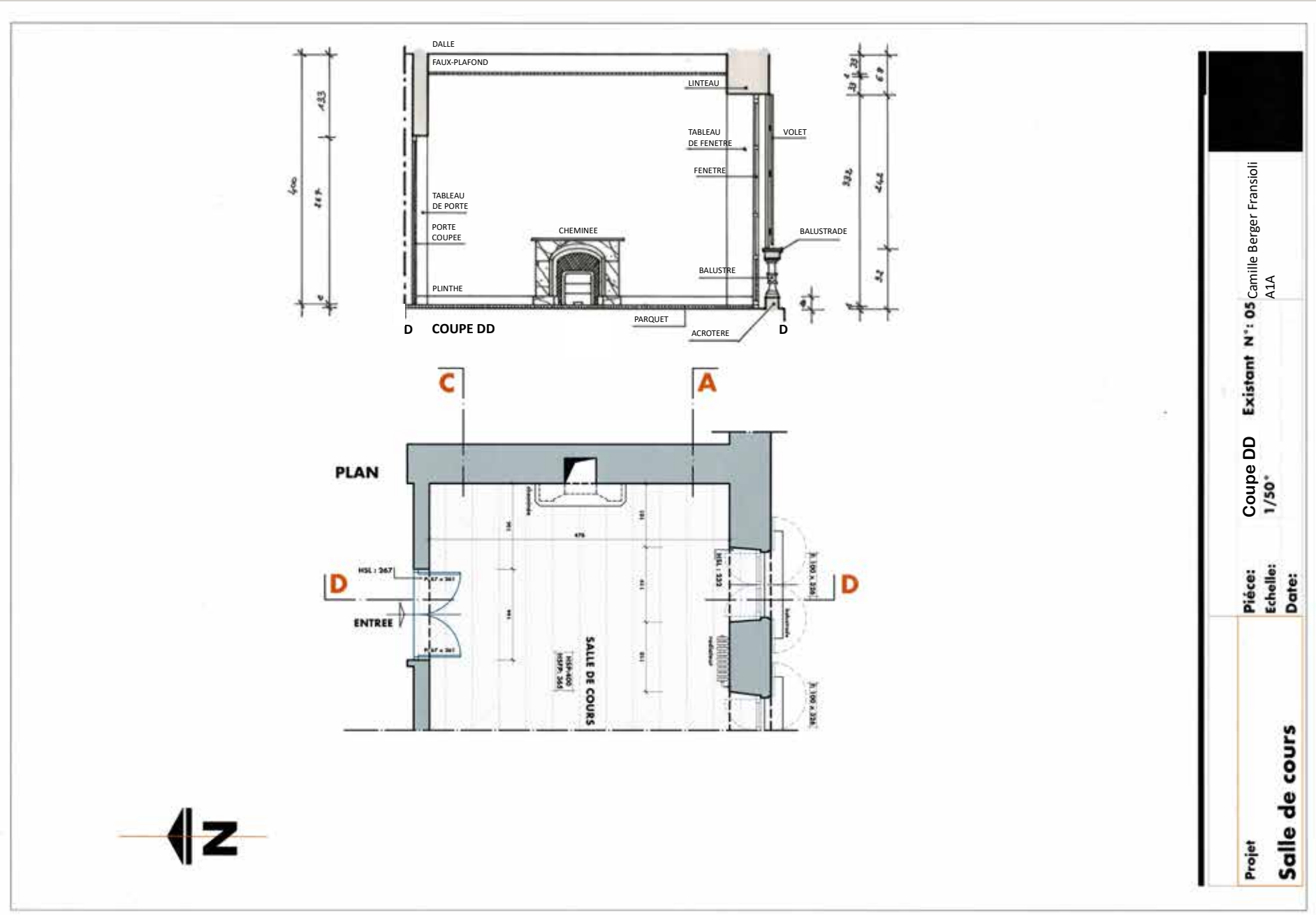
Salle de cours - Coupe DD réalisée au 1:50. Présentation Echelle N/C.
